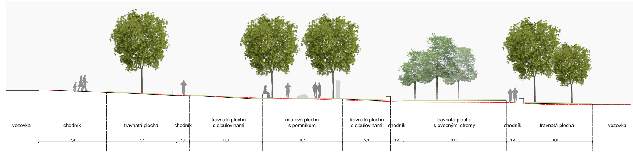
Řez F-F'
