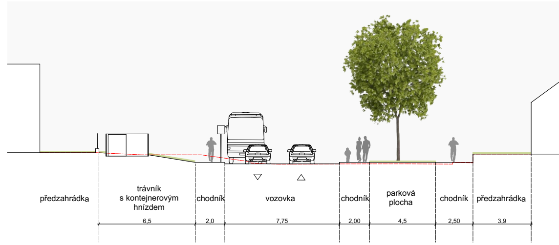
Řez A-A'
