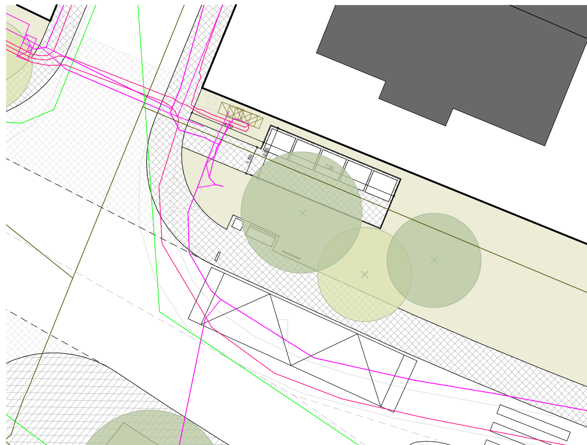
Varianta A - umístění kontejnerů na tříděný odpad podél plotu soukromé zahrady, za stávající elektro sloupky
