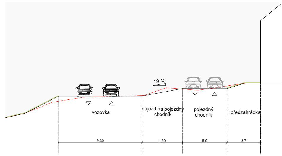
Řez E-E'
