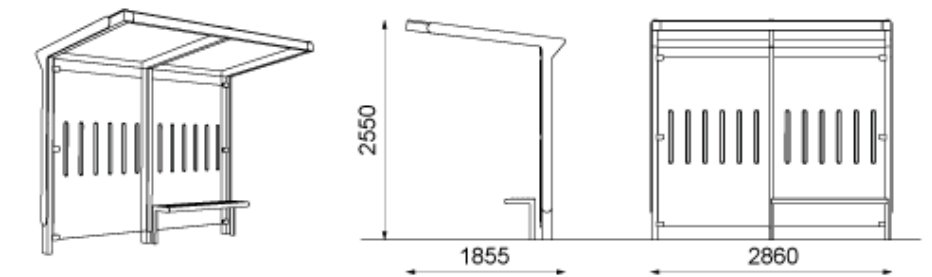
zastávkový přístřešek s plochou střechou mm-cite, aureo (AE200-LS)
