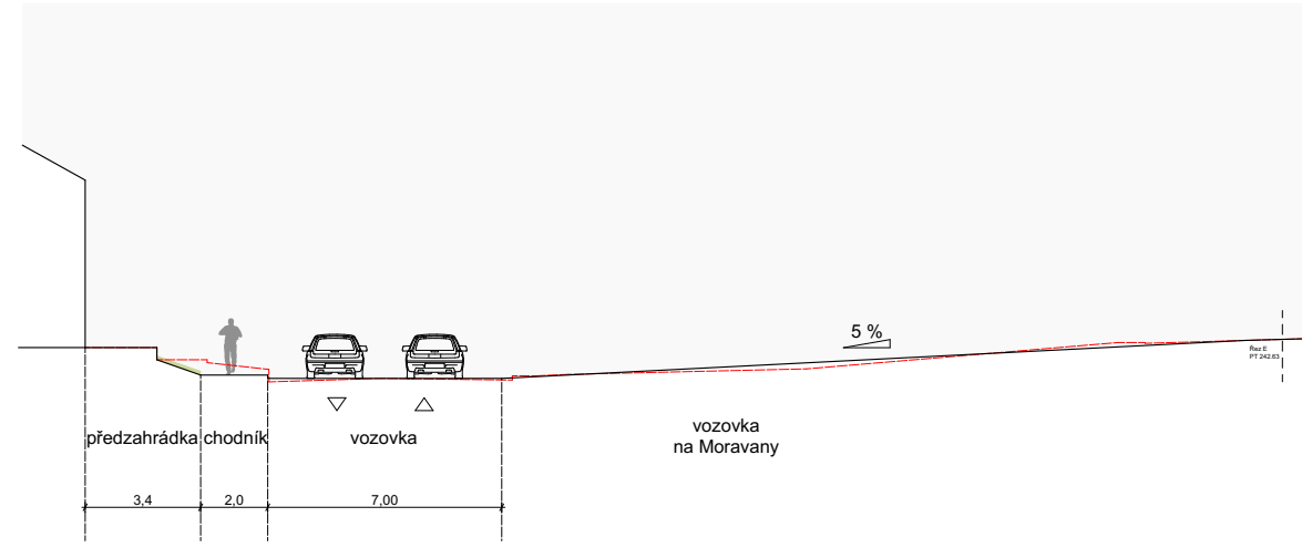
Řez D-D'
