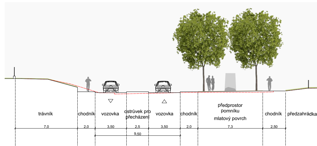
Řez B-B'
