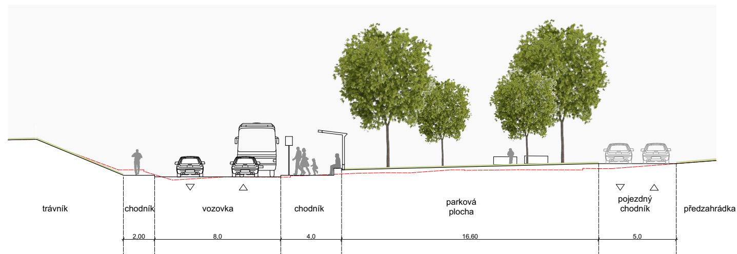
Řez C-C'
